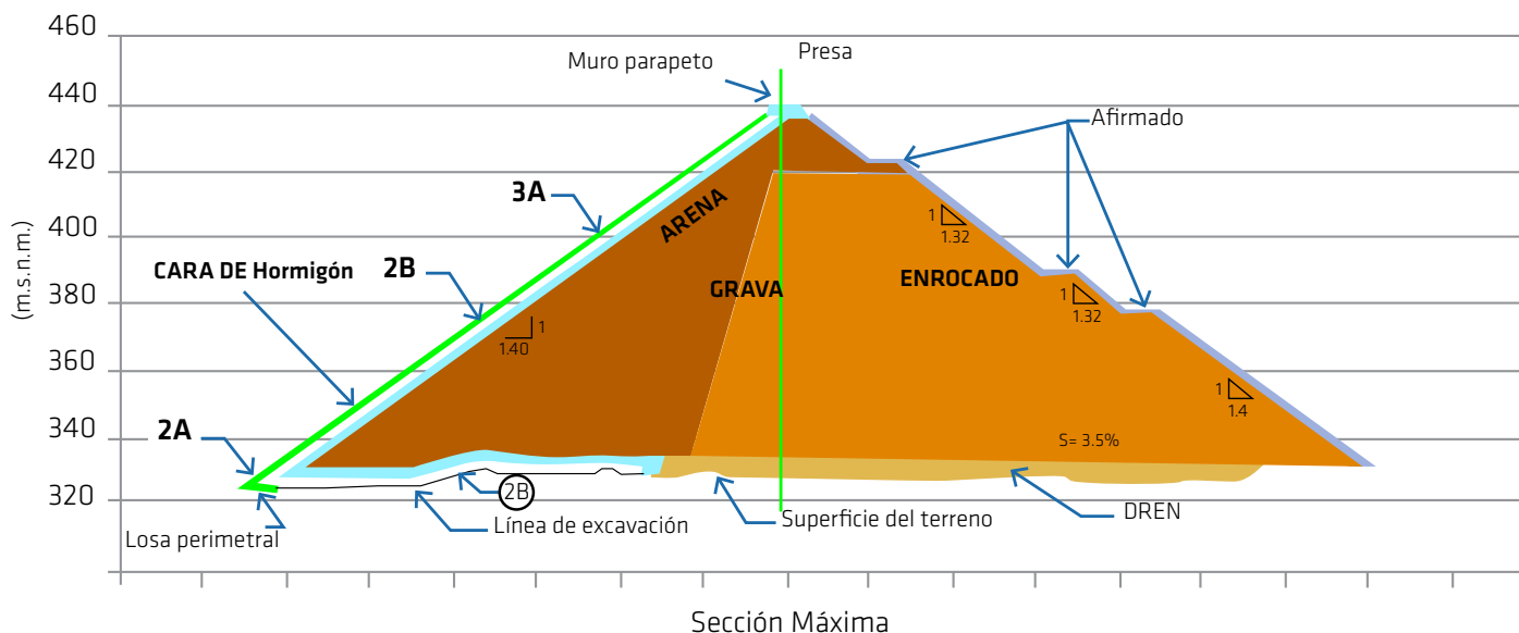
Figura 3. Esquema de una presa de enrocado y cara de hormigón (CFRD).
