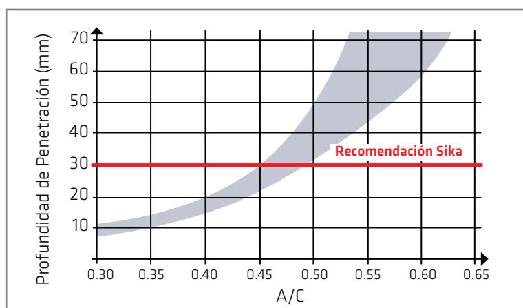
Figura 15. Relación entre la penetración de agua (mm) y la relación A/C de acuerdo con la norma EN 12390-8 [17]
