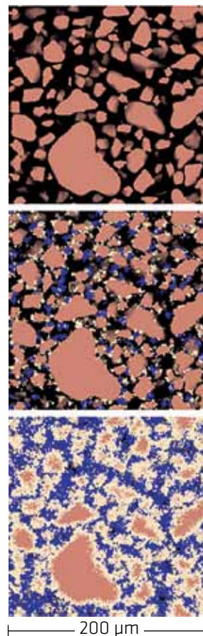
Figura 1. Modelación Jennings et al. (Bullard and Garboczi 2006) de una pasta de cemento ( C_3S ) A/C = 0.5 con diferentes grados de hidratación 0, 0.1 y 0.6 de arriba a abajo. En negro porosidad capilar, en café oscuro = C_3S y en café claro = C-S-H incluyendo los poros de gel, en azul Ca(OH)_2
