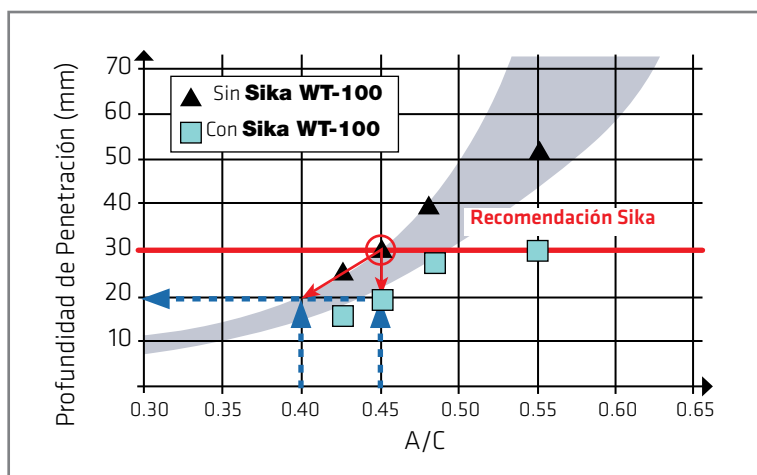
Figura 16. Resultados de Penetración de Agua vs. A/C superpuestos a resultados recientes LEM-Sika con y sin Sika WT100 [9] .
