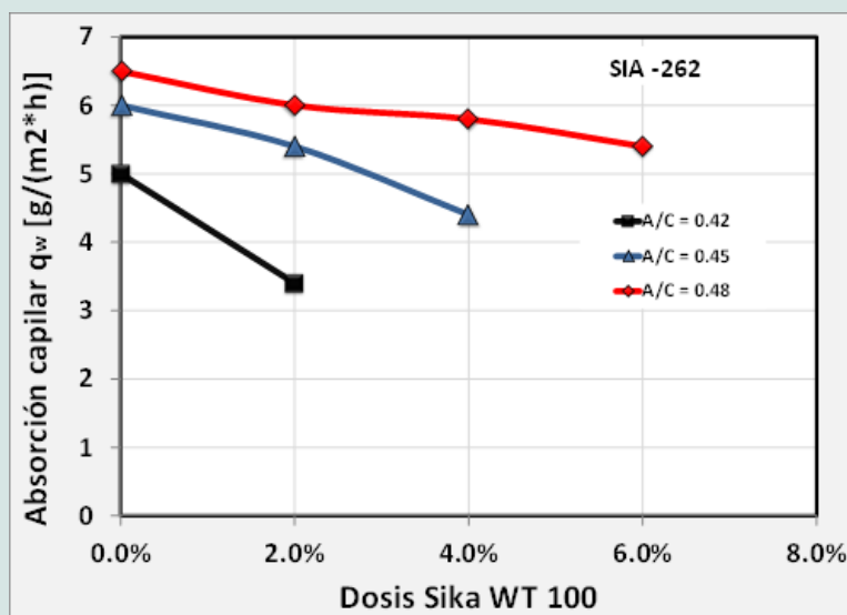
Figura 18. Efecto del aditivo Sika WT-100 para diferentes relaciones A/C y diferentes dosificaciones, frente a la penetración de agua por absorción capilar de acuerdo con la norma EN 262- Anexo A.
