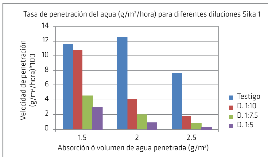
Figura 14. Velocidad de penetración de un volumen dado de agua por absorción capilar en morteros iguales que se diferencian solo por las concentraciones de Sika®-1 (Dilución de líquido de amasado de 1:10, 1:7.5, 1:5 – Aditivo:Agua)
