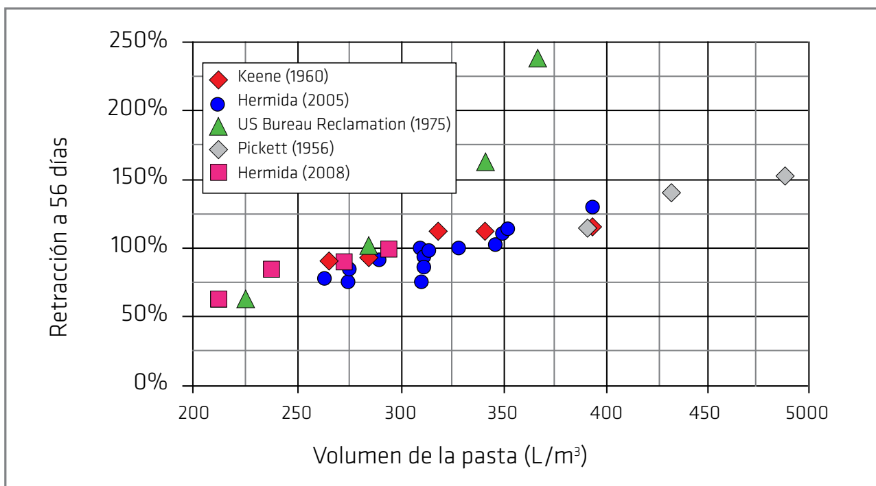
Figura 21. Relación entre el volumen de pasta y la retracción del hormigón [19] .
