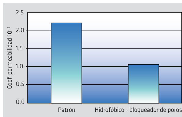
Figura 11. Efecto de la adición de un aditivo hidrofóbico en un hormigón con un coeficiente de permeabilidad de 1 \times 10^{-12} m/s
