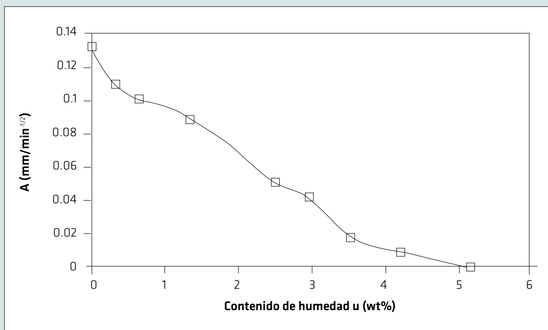
Figura 5. Efecto del contenido de humedad en hormigón sobre el coeficiente de absorción capilar (De Souza et al, 1998).
