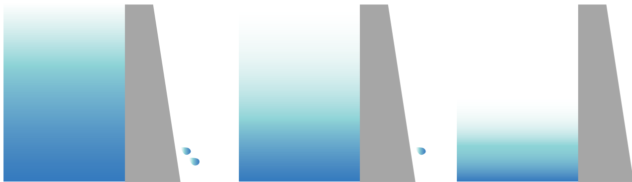
Figura 9. Influencia de la presión y área de contacto del agua sobre la filtración para estructuras de igual geometría, constituidas por la misma calidad de hormigón.
