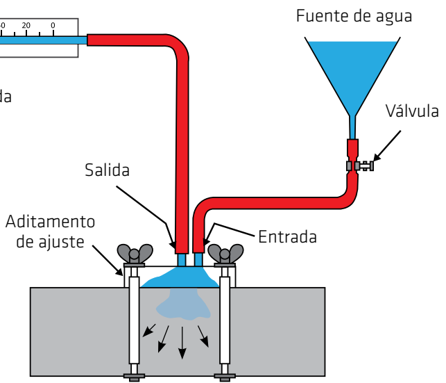
Figura 7. Ensayo de Absorción capilar ISAT-10 (Initial Surface Absorption Test-10 min) de acuerdo B5 1881
