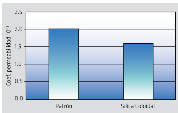
Figura 10. Efecto de la adición de sílica coloidal en un hormigón con un coeficiente de permeabilidad de 1 \times 10^{-13} m/s
