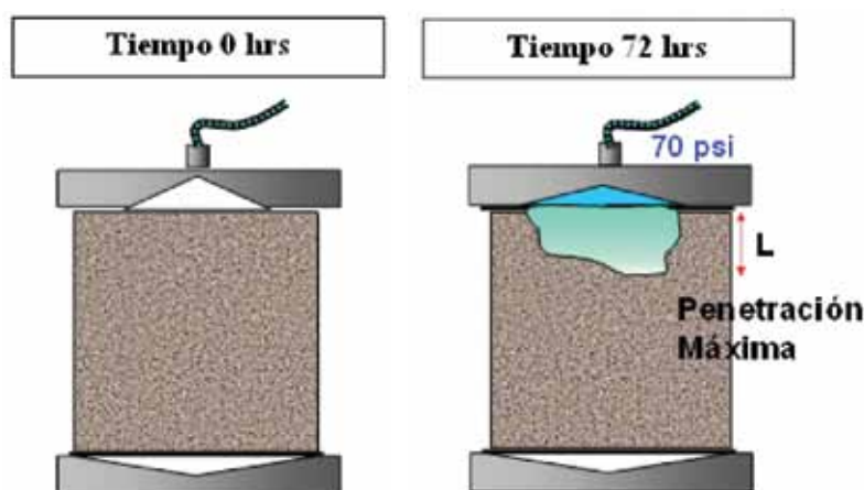
Figura 6. Esquema de funcionamiento de la norma EN 12390-8 de penetración de agua.
