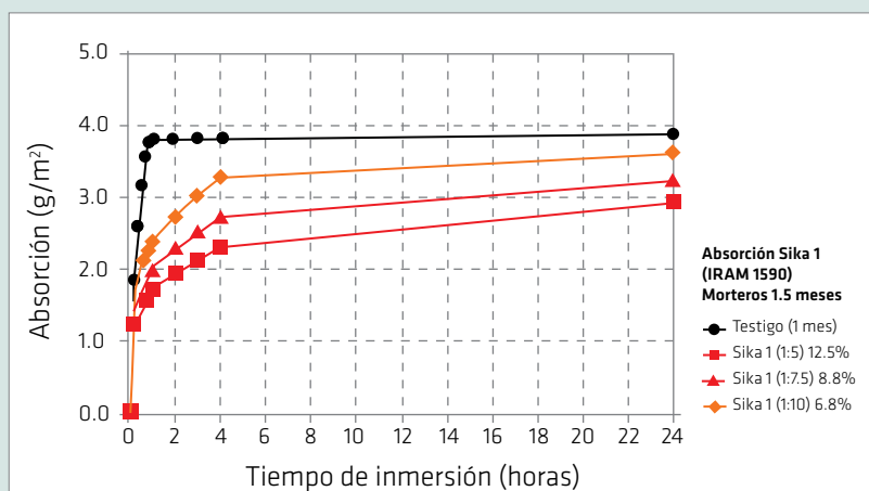
Figura 12. Efecto del Sika®-1 diluido a (1:5, 1:7.5 y 1:10- Sika®-1 : Agua) en un mortero de A/C = 0.75.
