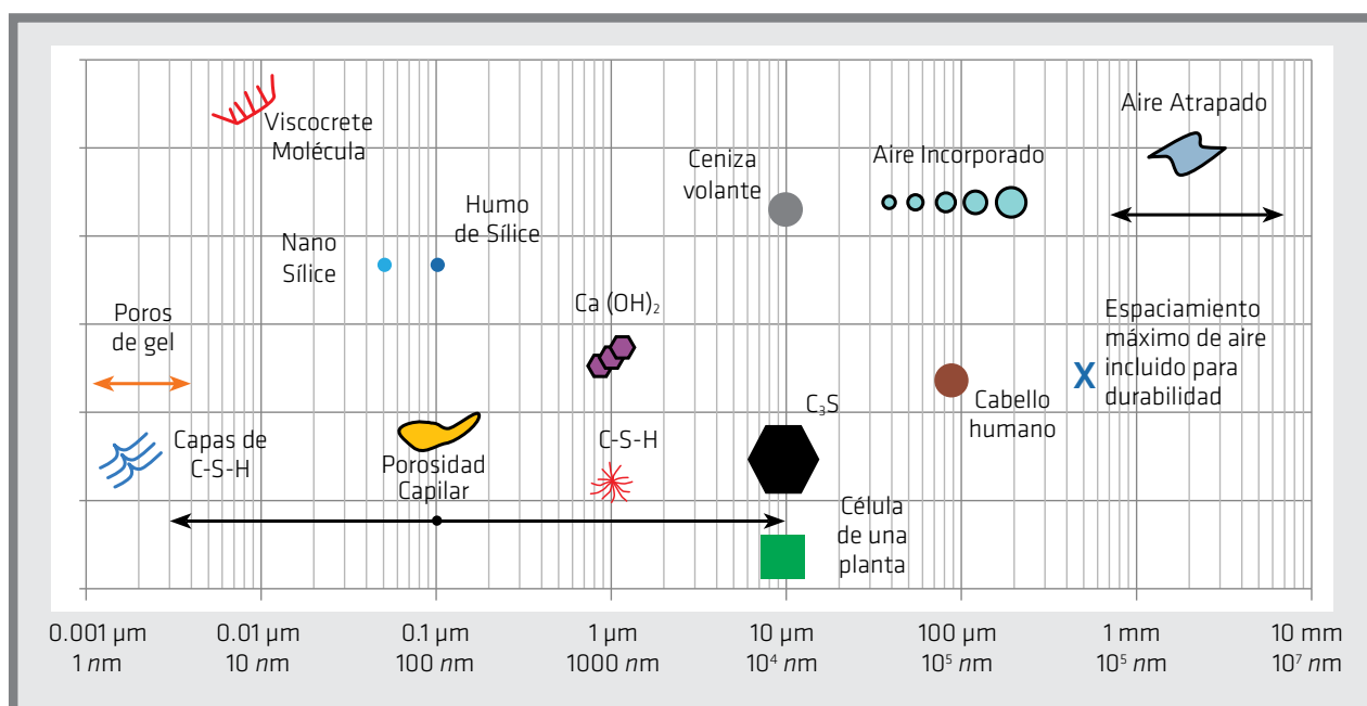
Figura 2. Escala de poros en el hormigón después de Mehta y Monteiro.
